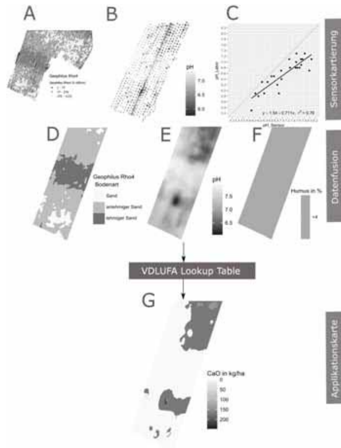
Abb. 4: Arbeitsschritte und Bodensensordaten zur Erstellung der Kalkapplikationskarte für das Versuchsfeld. (A) Geophilus ERA-Werte des Kanal 4 (0-100cm); (B) pH-Sensordaten der „on-the-go“-Messungen; (C) Regressionsmodell zur Kalibrierung der gemessenen Sensor-pH-Werte anhand von 25 pH[CaCl 2 ]-Referenzproben; (D) Räumliche Bodentexturverteilung auf Grundlage der Geophilus ERA-Werte des Kanal 4; (E) Interpolierte pH-Karte basierend auf den kalibrierten Sensordaten; (F) Humusgehalte liegen in der nach VDLUFA untersten Humusklasse (< 4%); (H) CaO-Applikationskarte in kg ha -1 basierend auf den fusionierten Sensordaten (Bodenart, pH, Humus) und der VDLUFA-Lookup-Table [Ri08].
